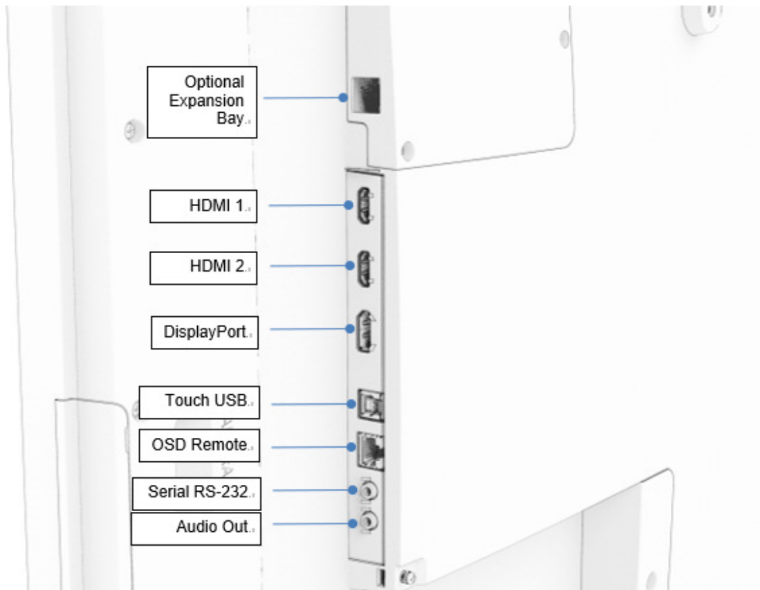
Porte I/O del display IDS
